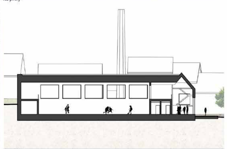
řez podélný
