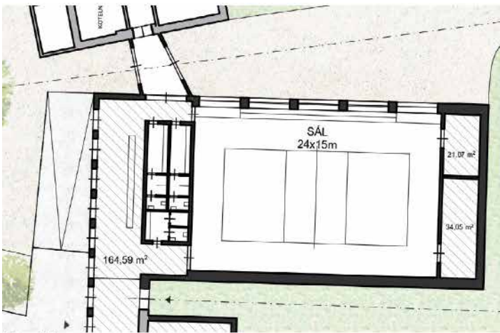
půdorys 1.NP
